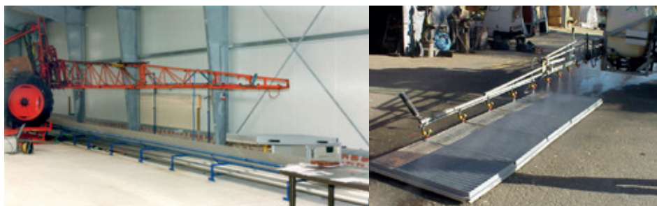
Fig. 18 : Équipements de mesure de la distribution d'une pulvérisation
