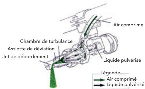
Fig. 11 : Buse à double fluide
