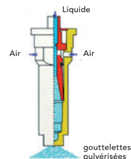
Fig. 12 : Buse à injection d'air
